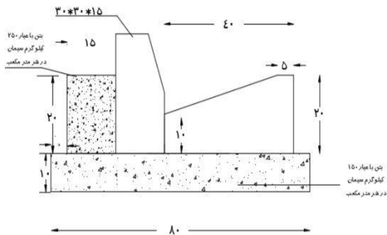
شکل ۵-۶- جزئیات نصب جداول کتابی - نوع B 2
