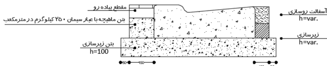
شکل ۵-۱۰- جزئیات نصب جداول آبروی کوتاه تیپ D
