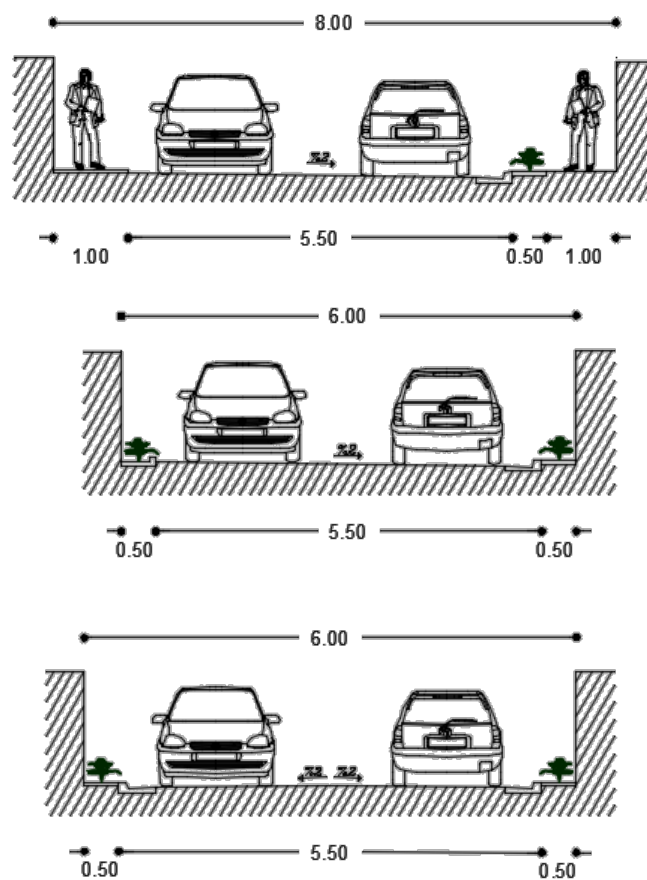
شکل پ ۲-۱۰-مقطع عرضی معبر تپ سه - عرض ۶ و ۸-کانیو نوع C
