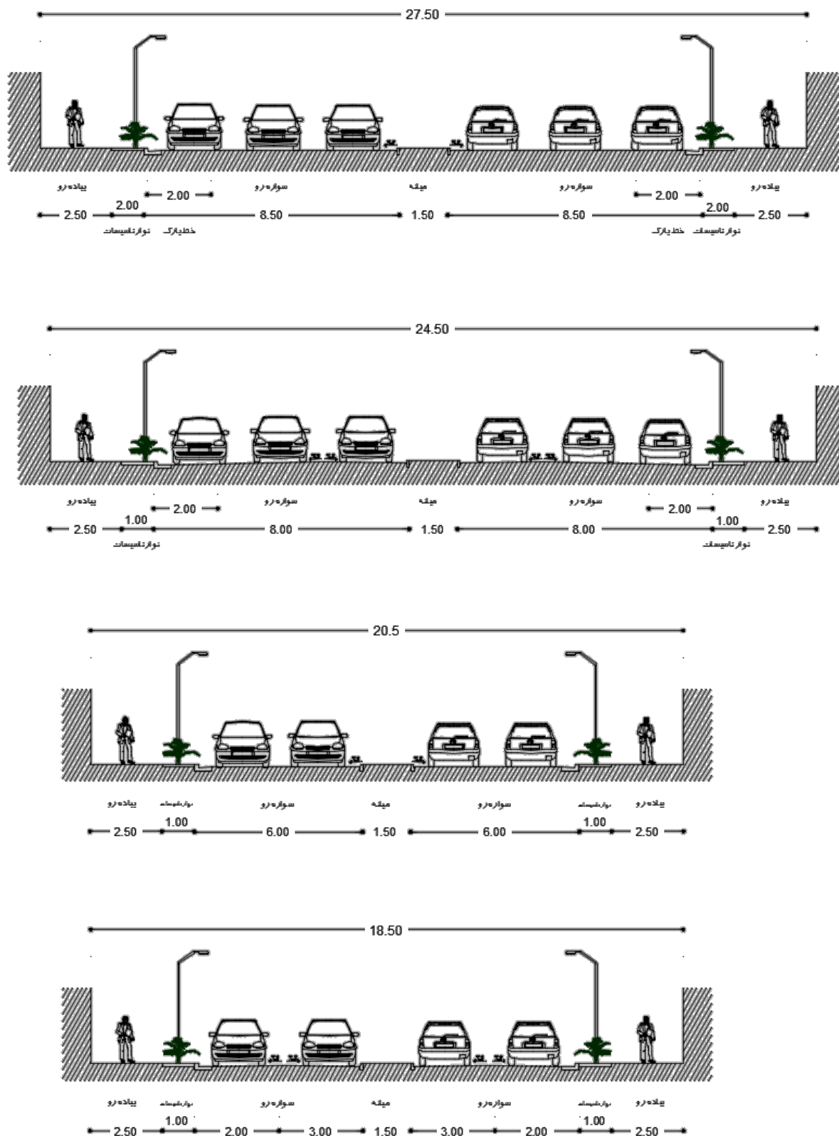
شکل پ ۲-۳-مقطع عرضی معبر تیپ یک - عرض ۲۷,۵، ۲۴,۵، ۲۰,۵ و ۱۸,۵- کانپو نوع D
