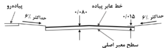
مقطع B-B
