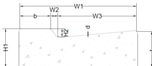
شکل ۵-۹- مشخصات ابعادی جداول آبروی کوتاه تیپ D
