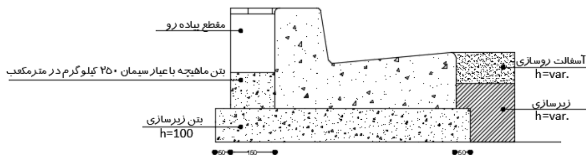
شكل ٥-٨- جزئيات نصب جداول نوع C
